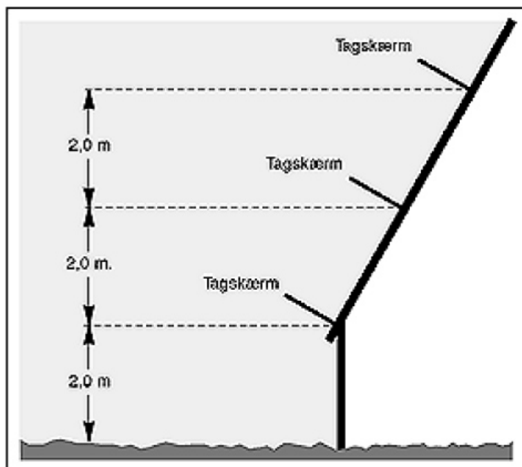
Fig. 5 Taghældning på 60 grader eller derover.
