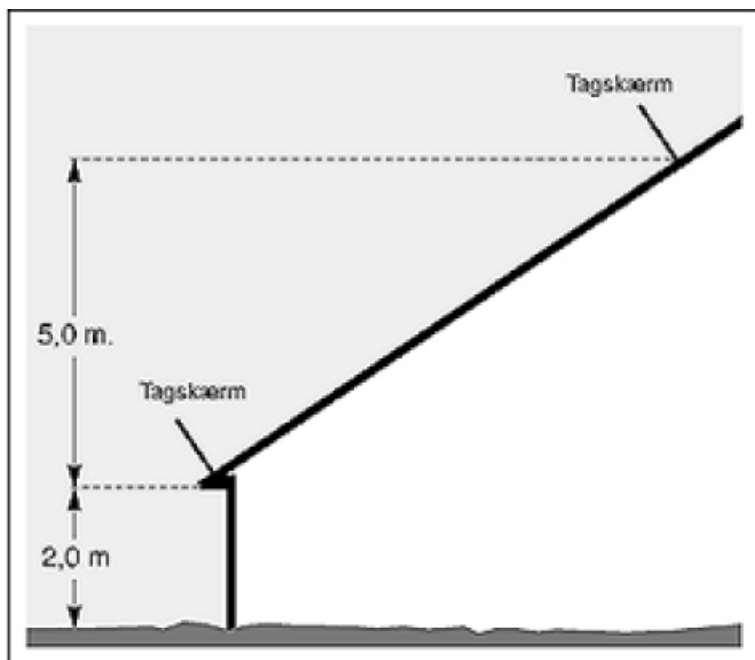
Fig. 4 Taghældning på 34 grader eller derover.
