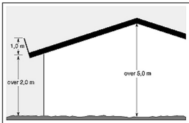
Fig. 3 Taghældning på 15 grader eller derover.
