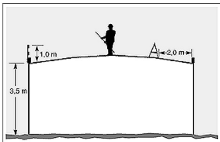
Fig. 2 Taghældning under 15 grader.
