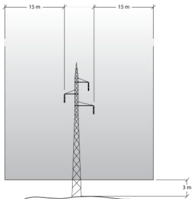
Figur 4 Højspændingsluftledninger 40-400 kV
