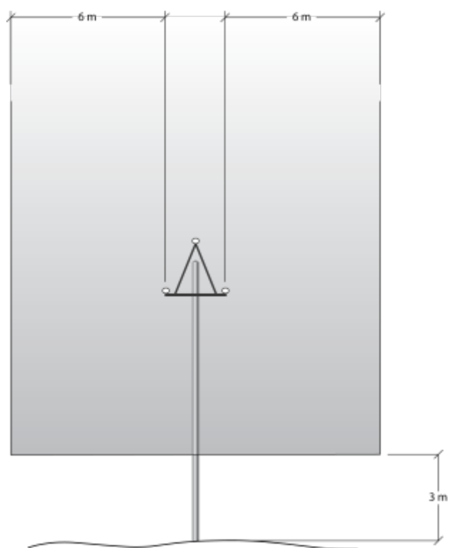
Figur 3 Højspændingsluftledninger 10-40 kV
