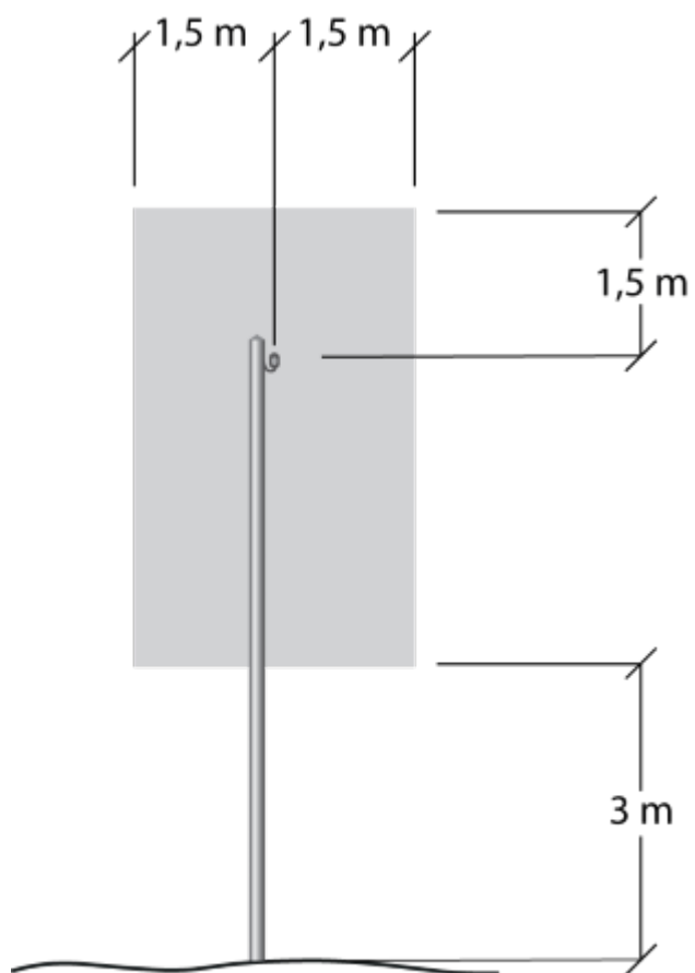
Figur 1 Lavspændingsluftkabler
