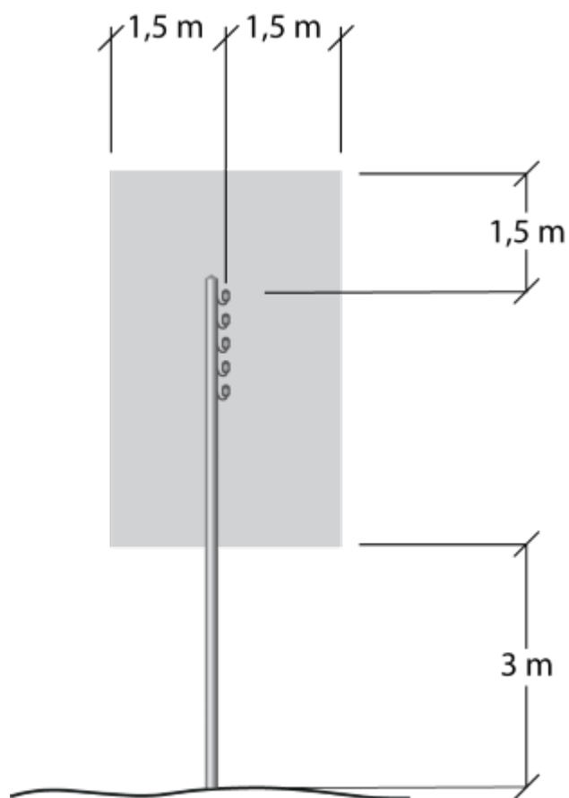
Figur 2 Lavspændingsluftledninger
