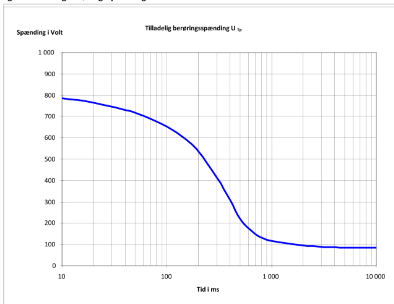
Figur 1 Tilladelig berøringspænding
