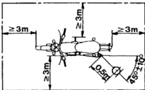
Mikrofonplacering og mindste måleplads
