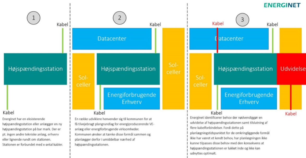
Figur: Principskitse over højspændingsstation, der lukkes inde ved placering af øvrige tekniske anlæg. Kilde: Energinet.
