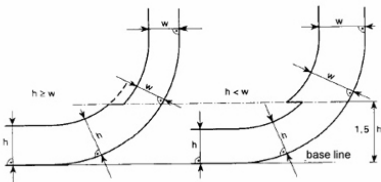
Figur 2 – Brændselsolietankens grænselinjer til brug for stk. 7 og 8
