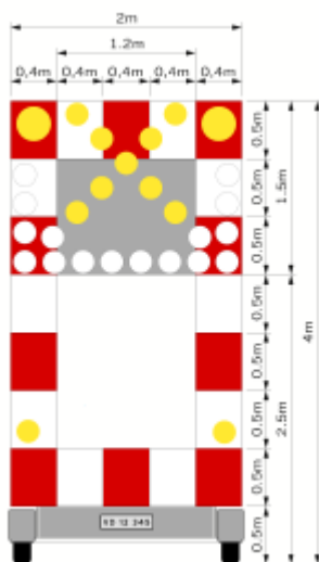
Figur 2. Afspærringsvogn med færdselstavle samt gule blinksignaler, der kan vise blinkende kryds eller pil orienteret mod højre eller mod venstre.
