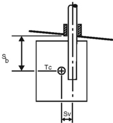
Skitse af spaderor
