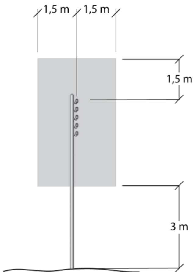
Figur 2 Lavspændingsluftledninger
