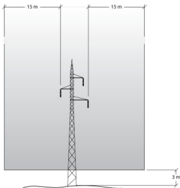
Figur 4 Højspændingsluftledninger 40-400 kV
