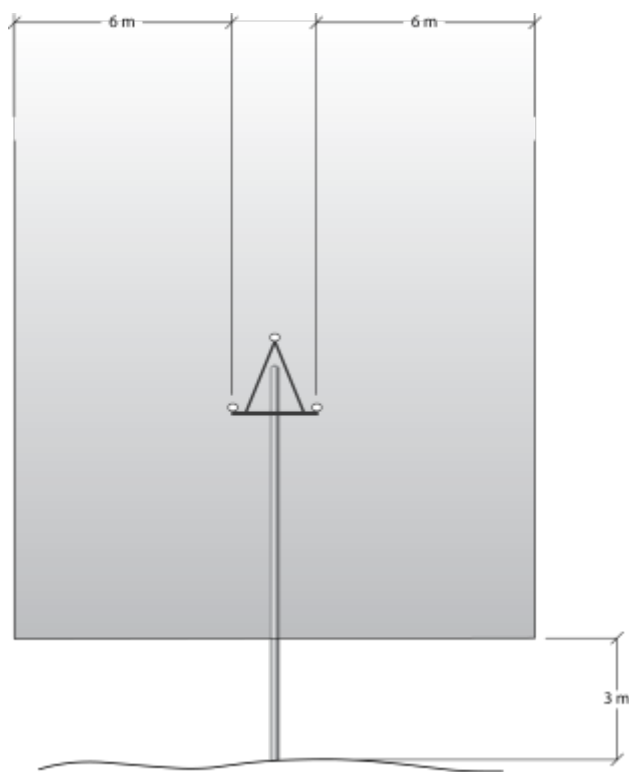
Figur 3 Højspændingsluftledninger 10-40 kV
