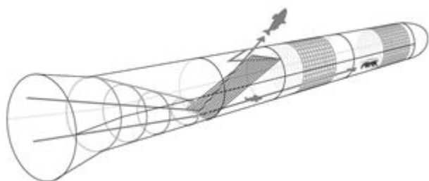
Figur 2. Illustration af et størrelses- og artsselektivt trawl, jf. nr. 2.
