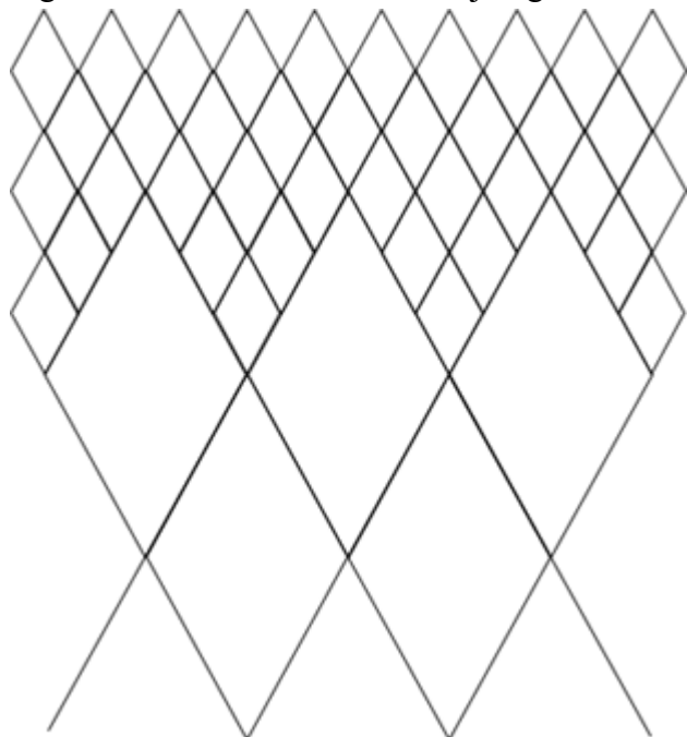
Figur 4. Illustration af sammenføjning af tre 90-100 mm. masker med én 270 mm. maske
