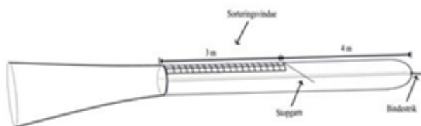
Figur 5. 2-panel fangstpose med et 180 mm kvadratmasket sorteringsvindue
