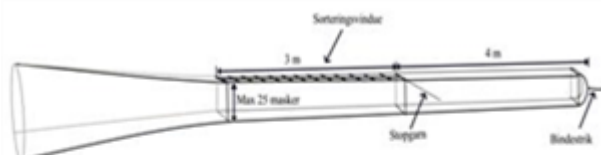
Figur 1. 4-panel fangstpose med et 180 mm kvadratmasket sorteringsvindue
