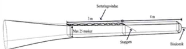
Figur 3. 4-panel fangstpose med et sorteringsvindue med diamantmasker på mindst 270 mm
