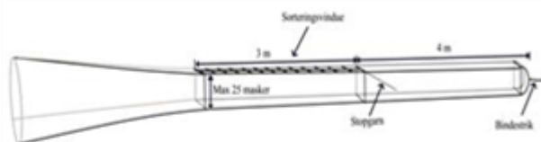
Figur 1. 4-panel fangstpose med et 180 mm kvadratmasket sorteringsvindue
