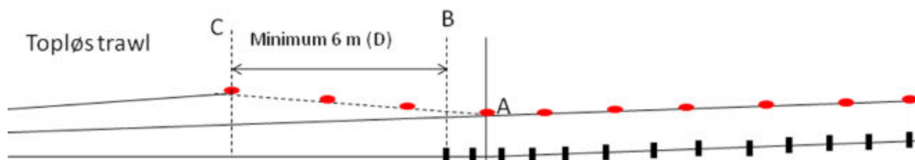
Fig 2. Skematisk tegning der illustrerer ændringen af en standard trawl til en topløs trawl set fra siden.
