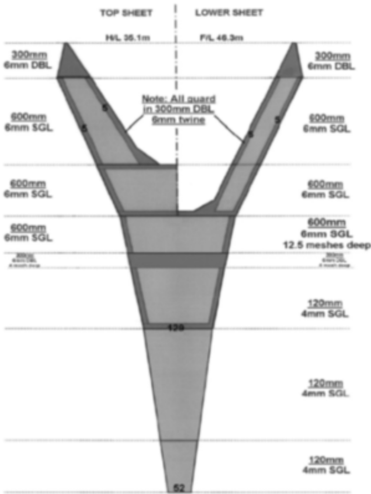
Figur 6: Oversigt over underpanel med mindstemaskestørrelse på 600 mm
