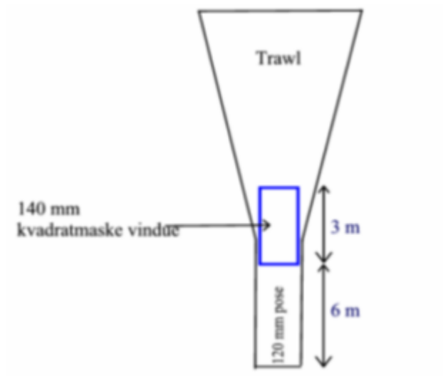
Figur 1: Skematisk tegning af 120 mm trawl og 140 mm panelets placering.
