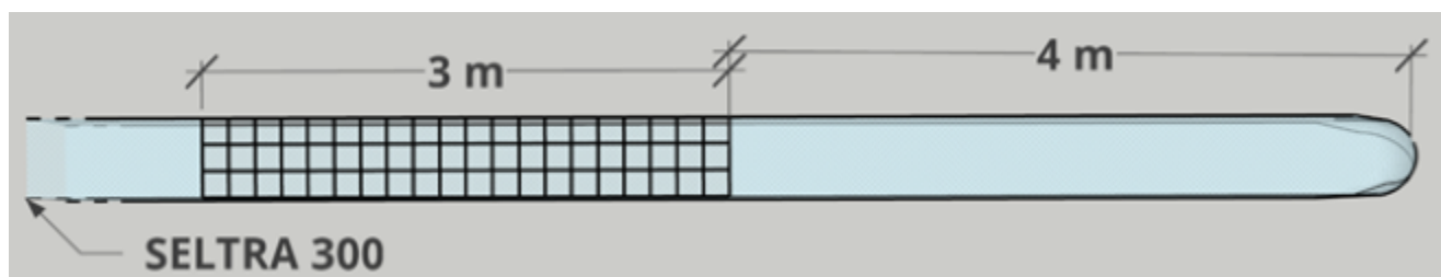
Figur 9: Seltrafangstpose med selektionsvinduet placeret 4 meter fra bindestrikken
