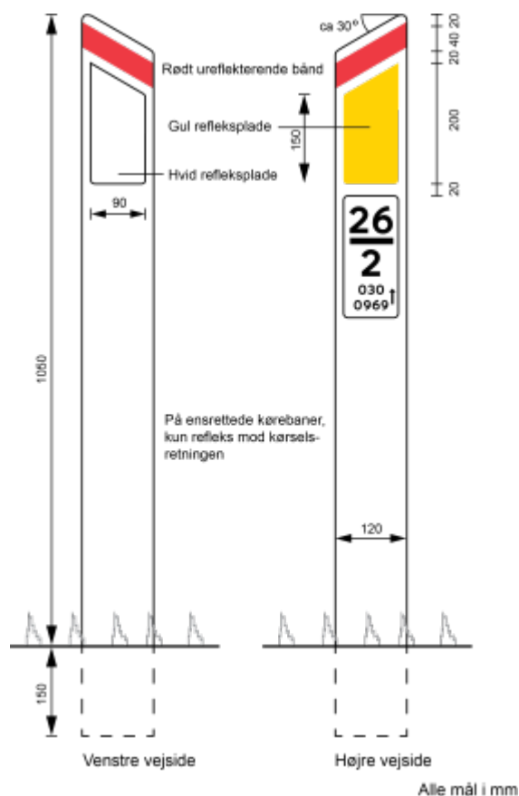
Figur 5. Kantpæl med kilometrerings
