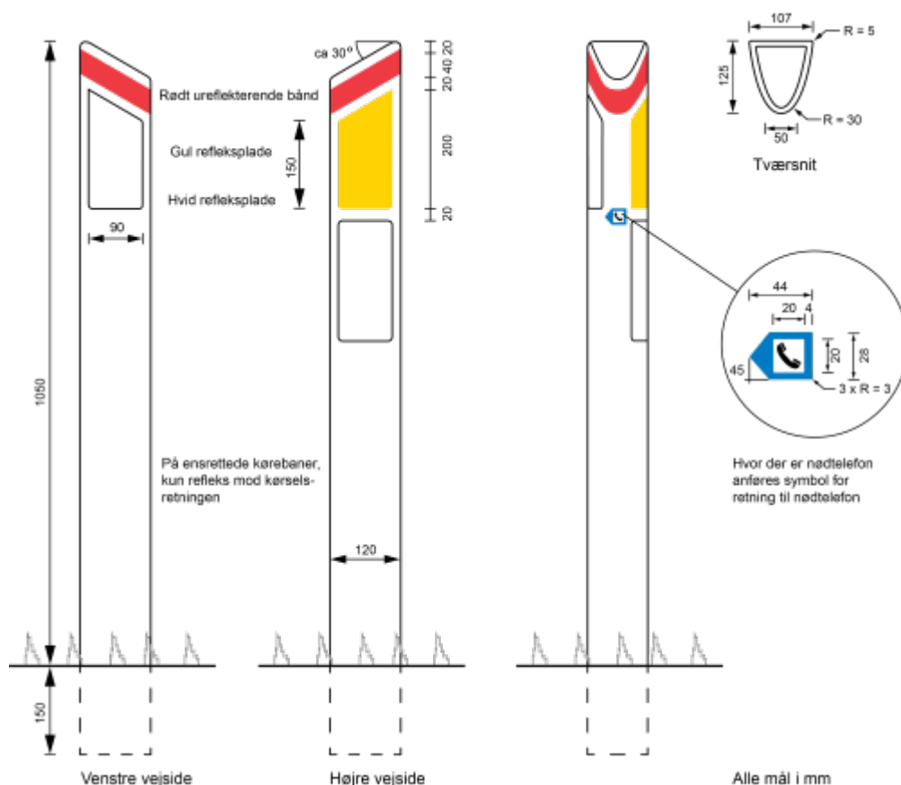
Figur 1. Kantpæl
