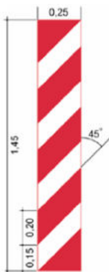
Figur 3. N 42 Kantaafmærkningsplader
