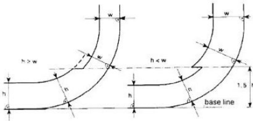
Figur 2 – Brændselsolietankens grænselinjer til brug for stk. 7 og 8
