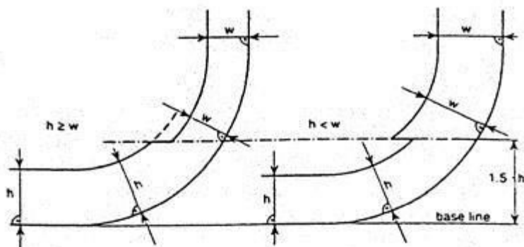
Figur 1 - Lasttankenes grænselinier jf. stk. 3
