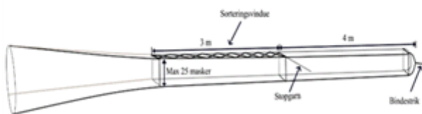
Figur 3. fire-panel fangstpose med et selektionspanel med diamantmasker på mindst 270 mm
