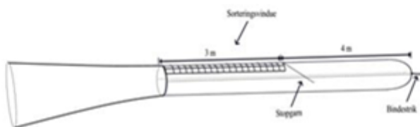
Figur 5. To-panel fangstpose med et 180 mm kvadratmasket selektionspanel
