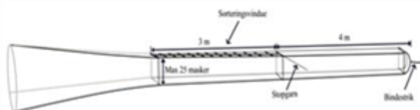
Figur 1. fire-panel fangstpose med et 180 mm kvadratmasket selektionspanel
