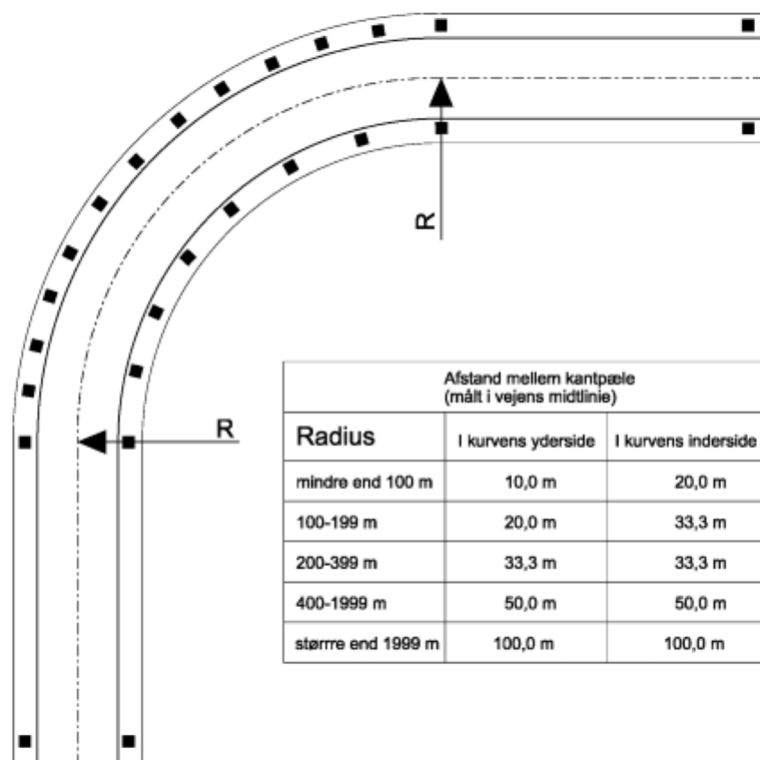
Figur 2. Placering af kantpæle i kurver
