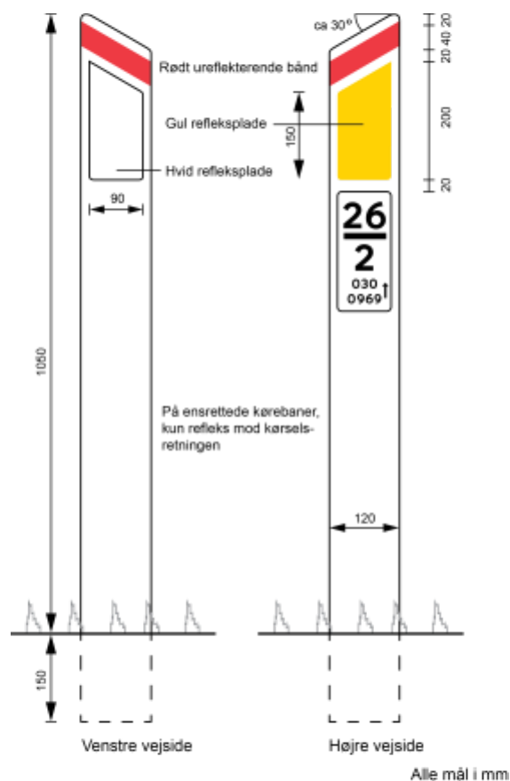
Figur 5. Kantpæl med kilometrering
