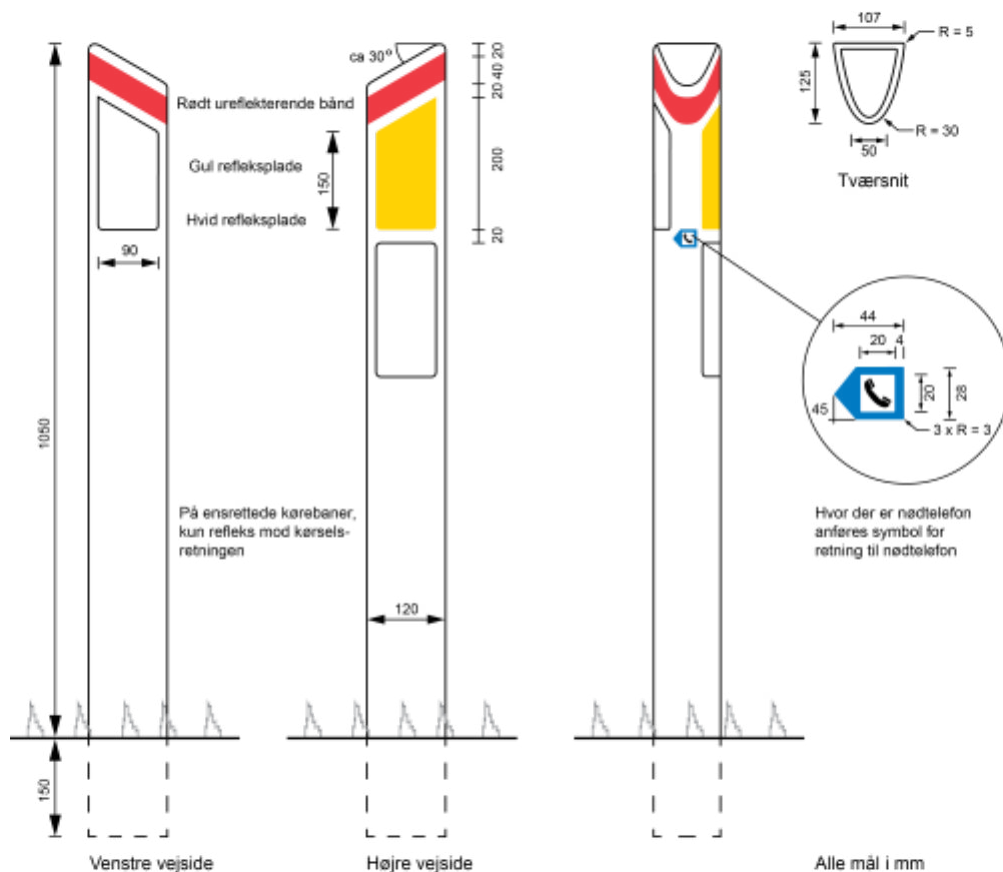
Figur 1. Kantpæl
