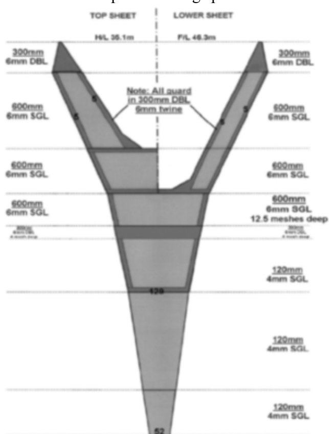
Figur 6: Oversigt over underpanel med mindstemaskestørrelse på 600 mm
