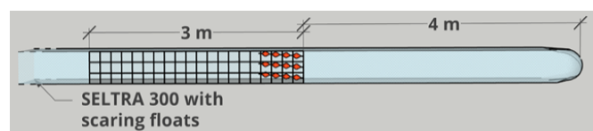
Figur 2: Seltrafangstposen med skræmmekugler og selektionsvindue
