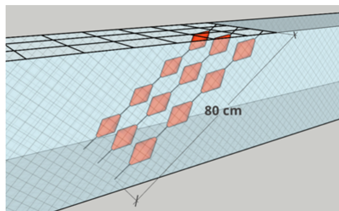
Figur 3: Placering af skræmmekugler i Seltrafangstposen
