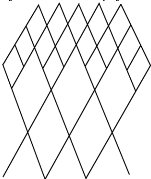
Figur 6. Illustration af sammenføjning af tre 90 mm. masker med én 140 mm. maske.
