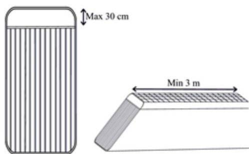
Figur 2. Illustration af et størrelses- og artsselektivt trawl, jf. nr. 2.
