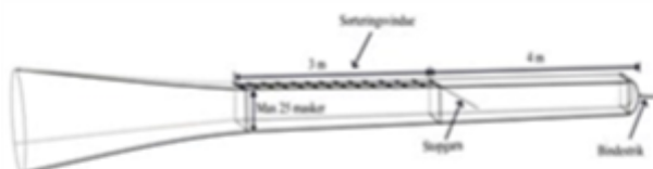
Figur 1. fire-panel fangstpose med et 180 mm kvadratmasket selektionspanel
