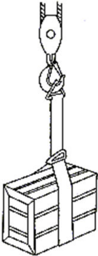
Fig. 21 Kunstfiberstrop
