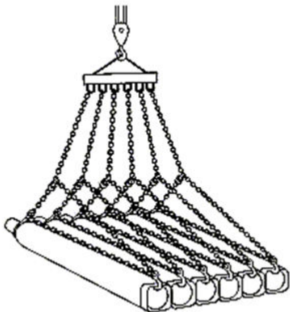
Fig. 35 Løft af flere trykflasker
