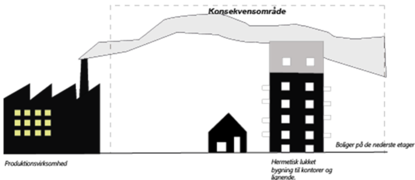
Fig. 9. Eksempel på planlægning på arealer belastet af lugt, støv og anden luftforurening ved brug af afskærmningsforanstaltninger. Den øverste del af etagebyggeriet, som rammes af en forureningsfane fra en produktionsvirksomhed, er hermetisk lukket med mekanisk ventilation. Der kan være kontorerhverv på de øverste lukkede etager. På de øvrige etager, hvor der ikke er en forureningsfane, kan der etableres boliger med altaner.
