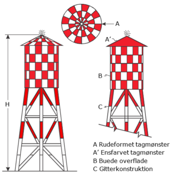
Figur 2-3: Eksempel på dagafmærkning og natafmærkning
