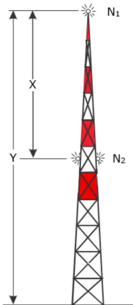
Figur 2-1: Dagafmærkning og placering af hindringslys
