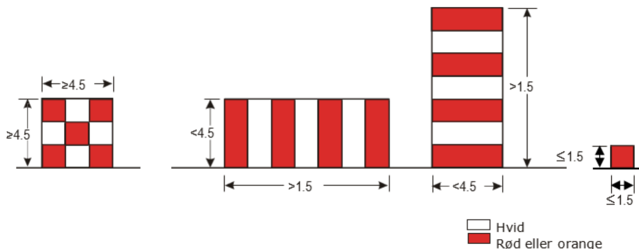
Figur 15-5 Grundlæggende afmærkning af luftfartshindringer med farver
