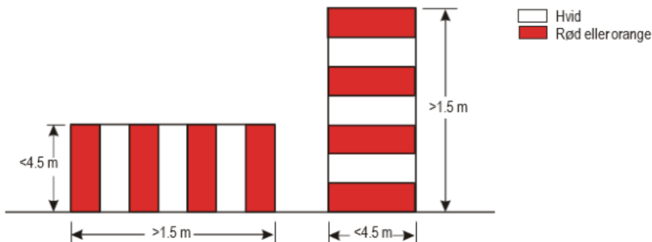
Figur 10-1: Grundlæggende afmærkning af luftfartshindringer med farvebånd
