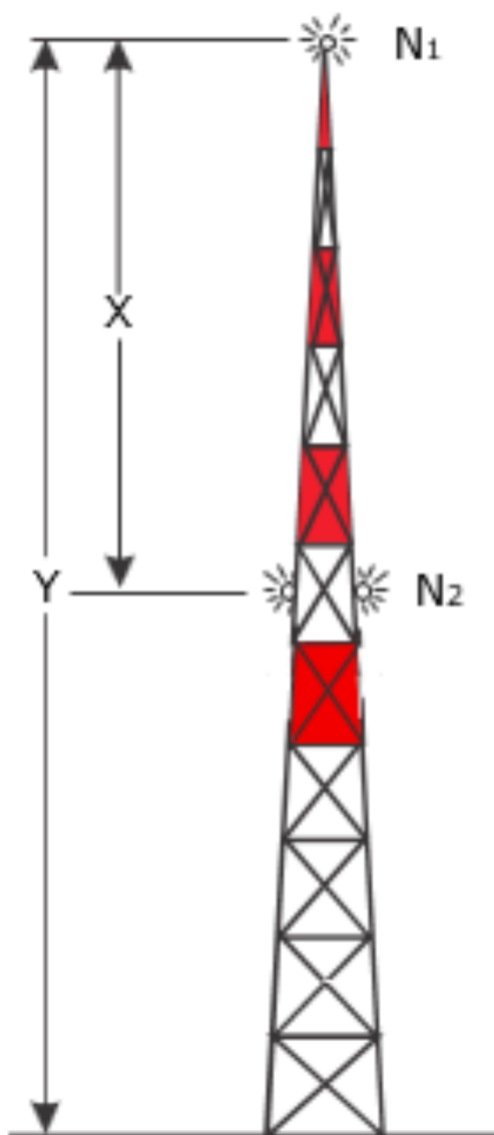
Figur 18-1: Dagafmærkning og placering af hindringslys
