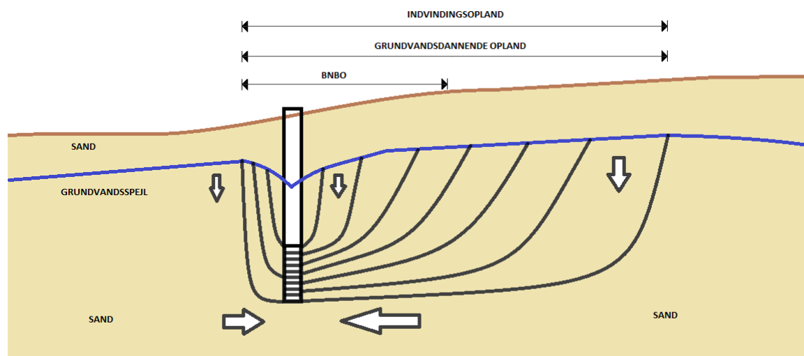
FIGUR 5. Illustration af et BNBO i et frit sandmagasin uden dæklag 7) .
